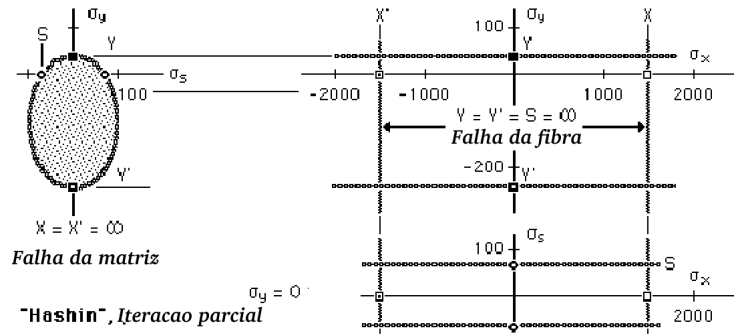
Figura 9.7: Três vistas do critério de Hashin (T300/5208).
